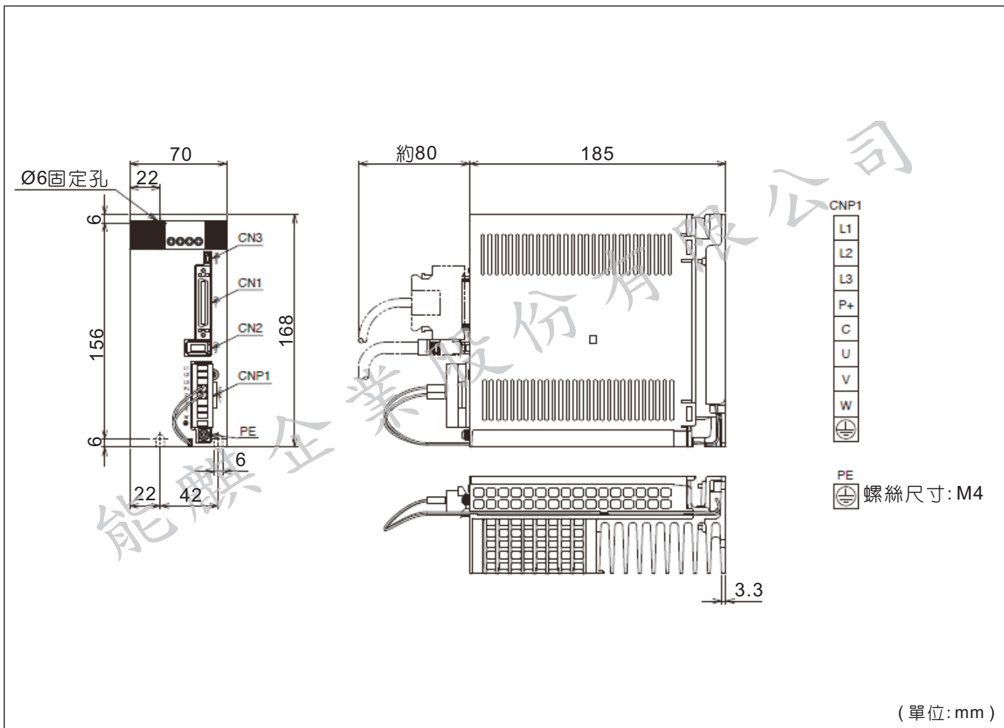
三菱電機MR-JE-70A、MR-JE-100A伺服驅動器外型尺寸圖
