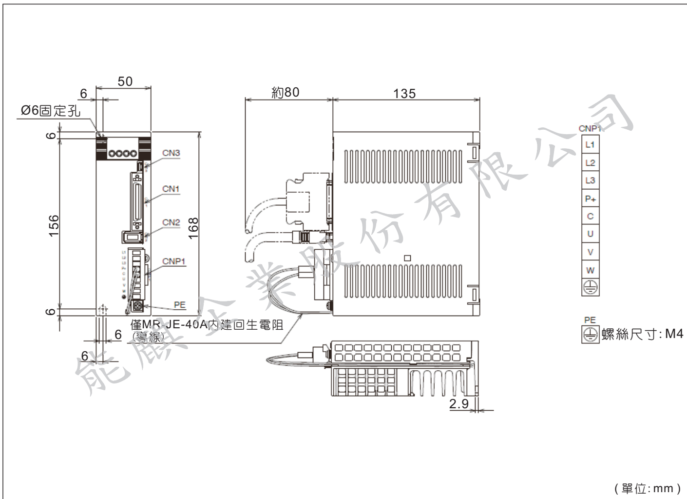
三菱電機MR-JE-10A、MR-JE-20A、MR-JE-40A伺服驅動器外型尺寸圖
