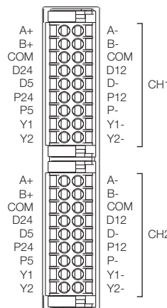
FX5-2HC/ES
