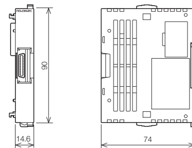
FX5-CNV-IFC
