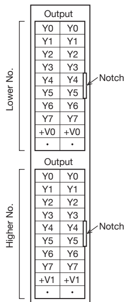
FX5-C32EYT/DSS
