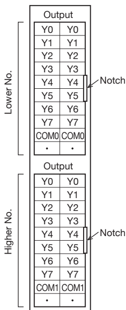
FX5-C32EYT/D
