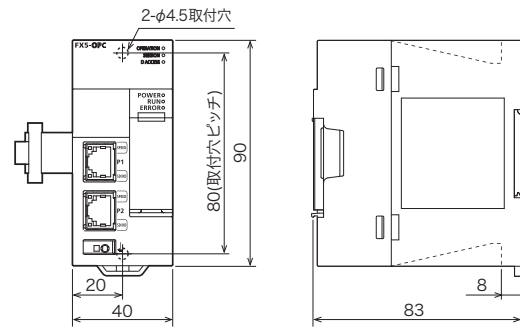
FX5-OPC
