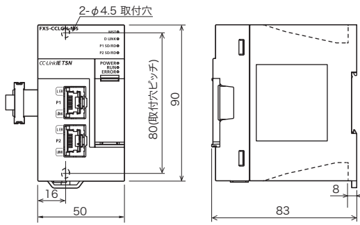
FX5-CCLGN-MS
