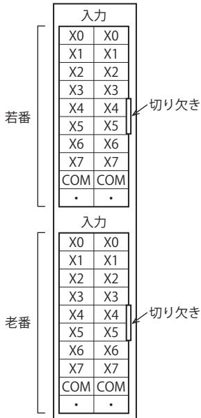
FX5-C32EX/D
