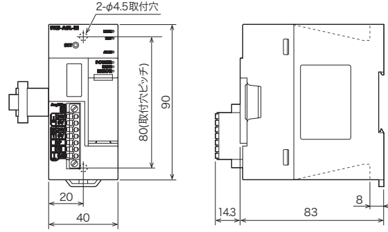
FX5-ASL-M
