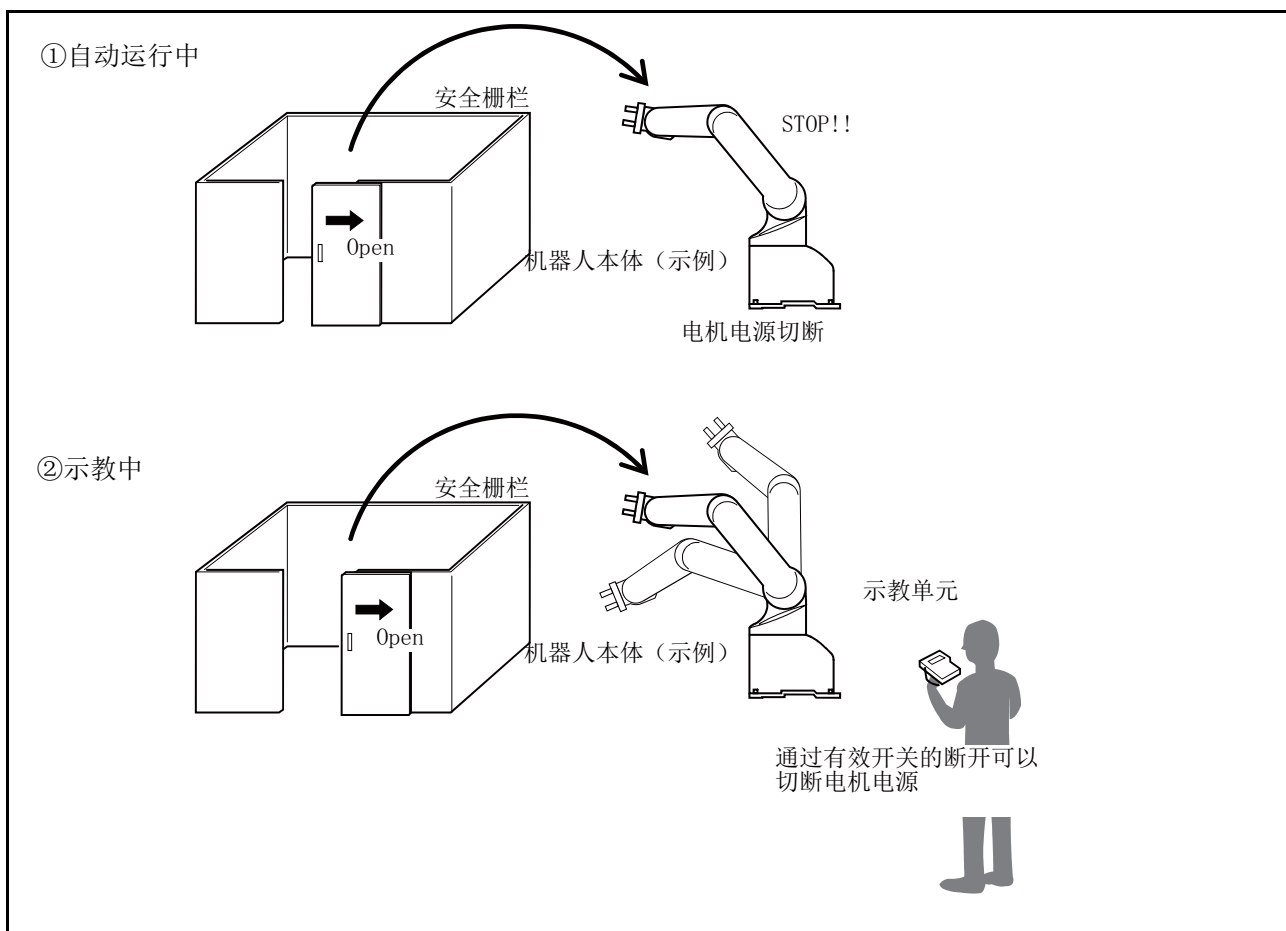
图 3-11：门开关的功能
