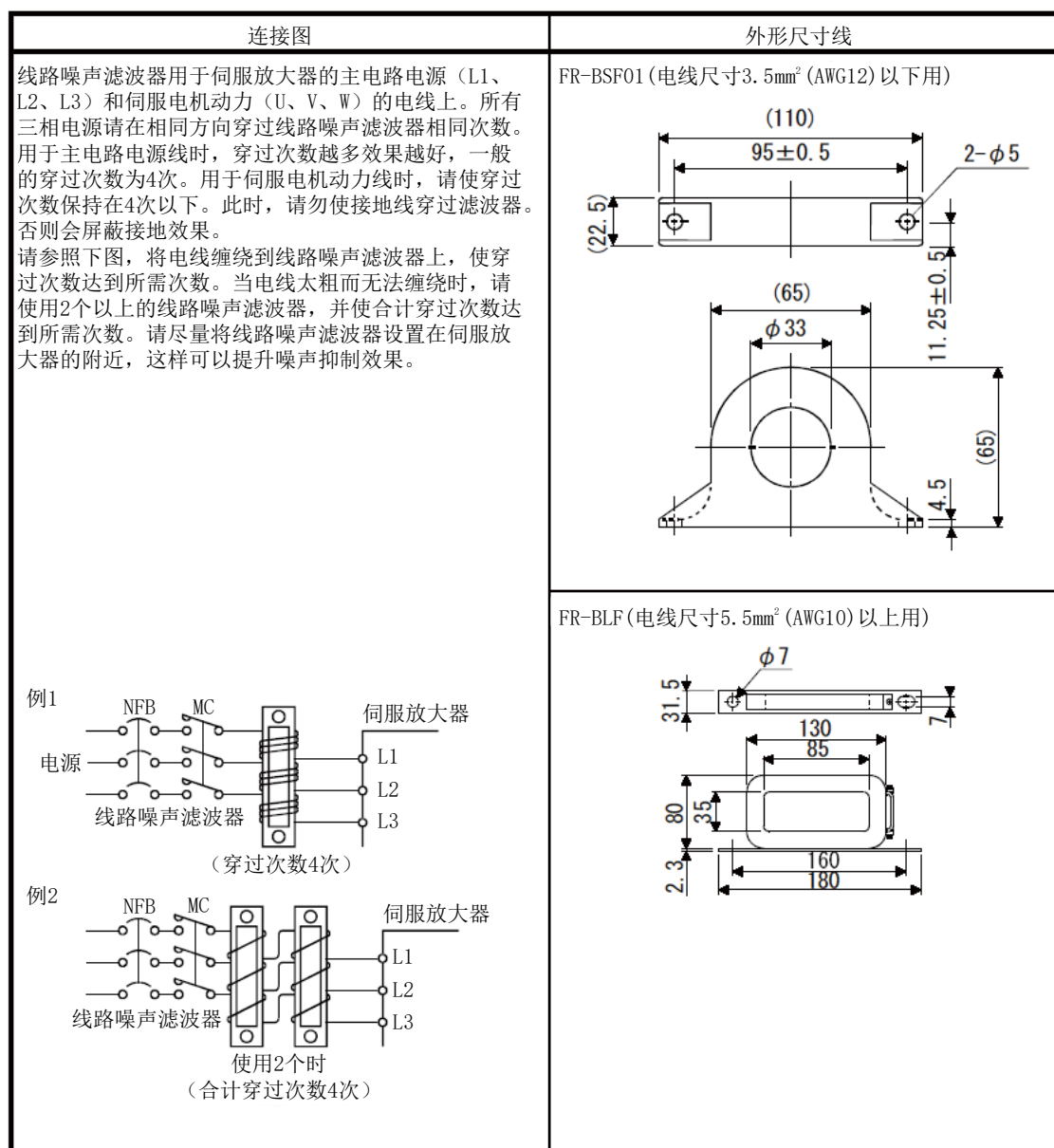
图 3-15：噪声滤波器的安装示例
