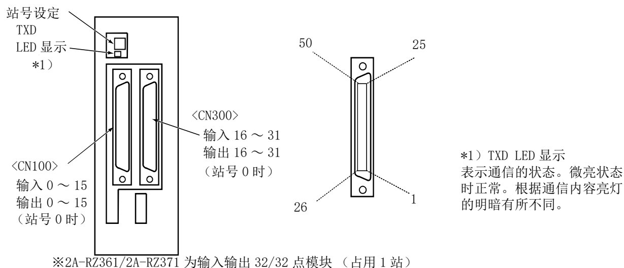
图 3-31: 并行输入输出模块的连接器针配置
