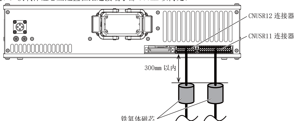
图 3-6: 铁氧体磁芯的安装位置
