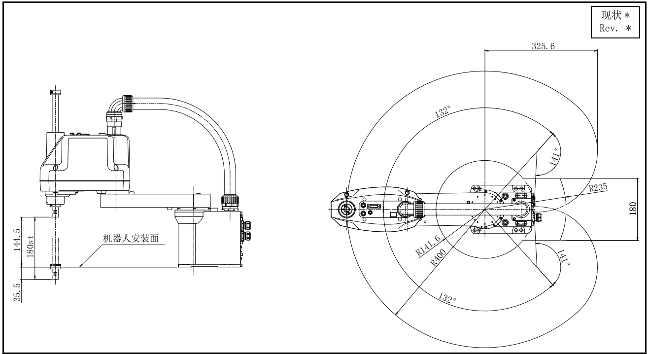
图 2-11: RH-3CRH4018 动作范围图
