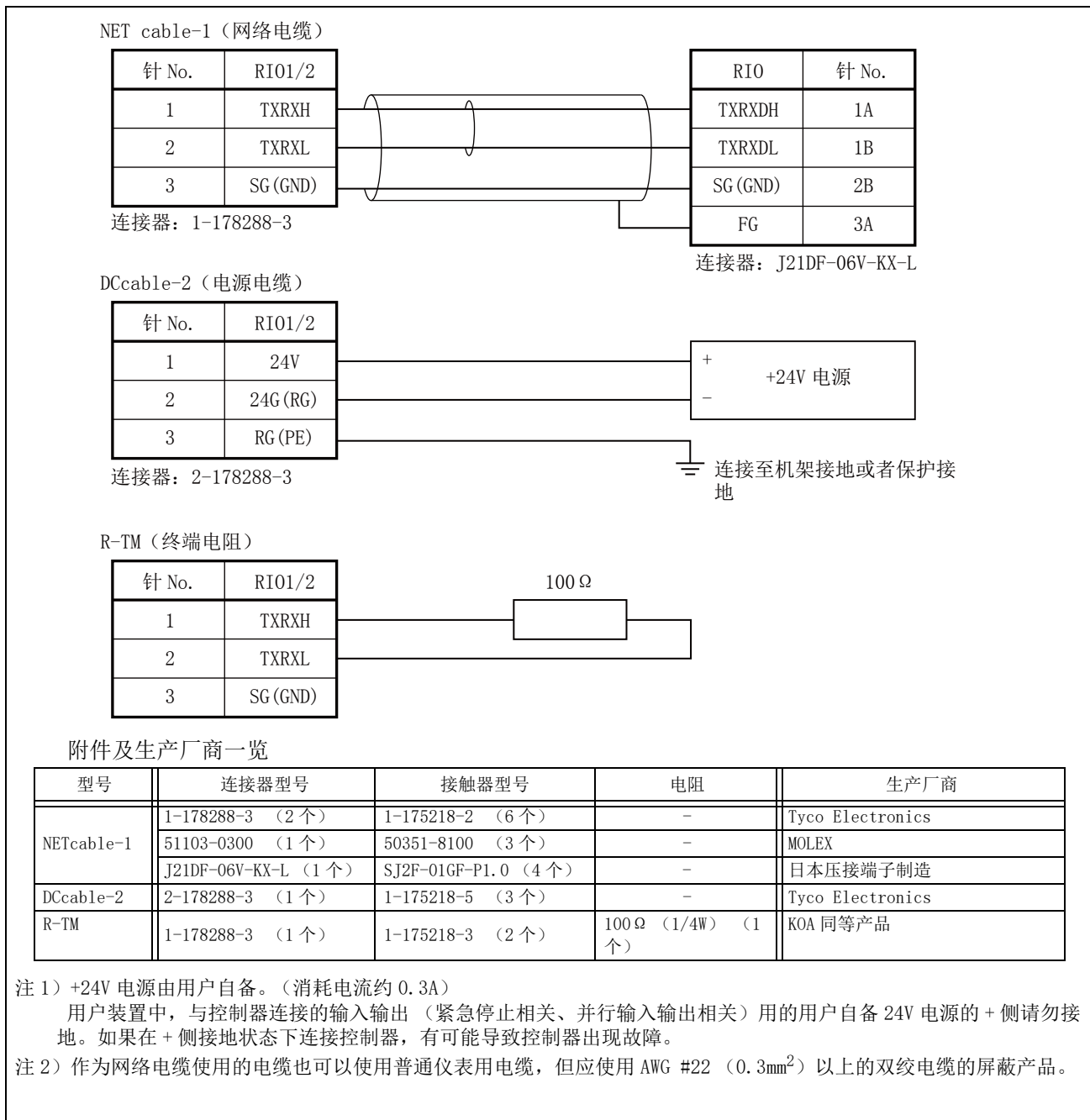
图 3-28: 连接电缆的规格
