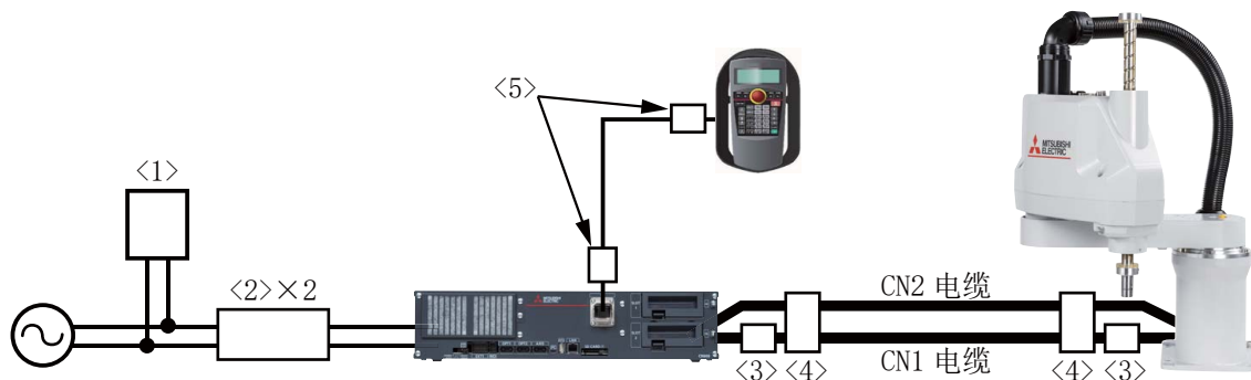
图 6-5：EMC 对策具体示例
