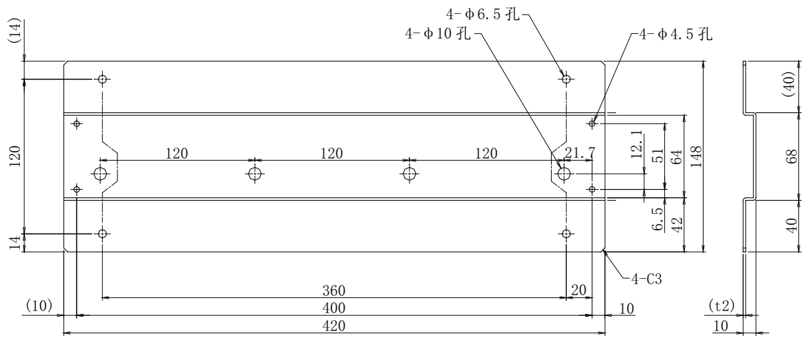
图 3-4：纵向安装用固定薄板参考图
