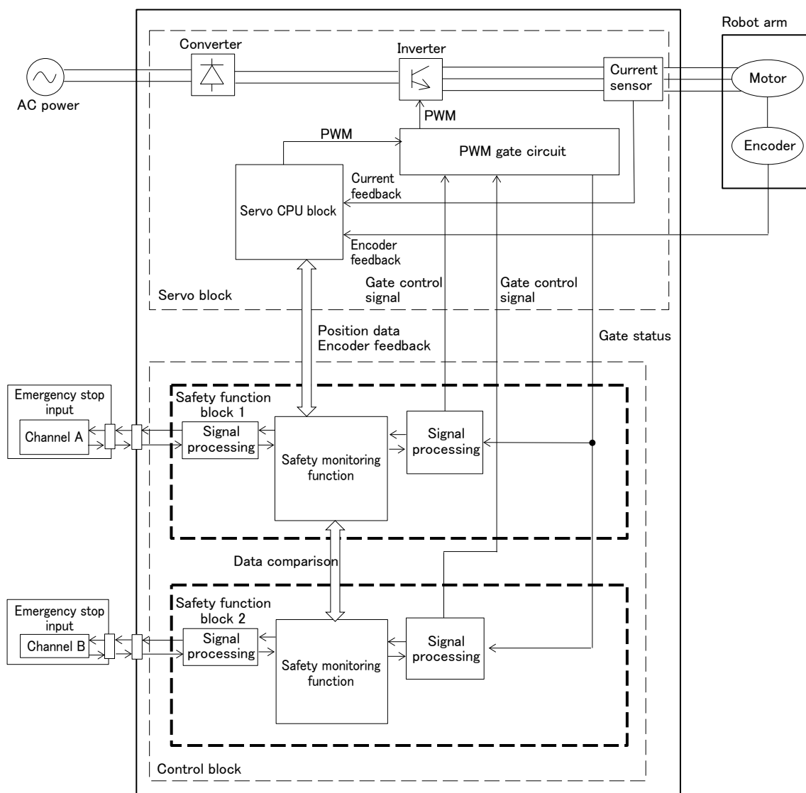
图 7-3: 安全块图
