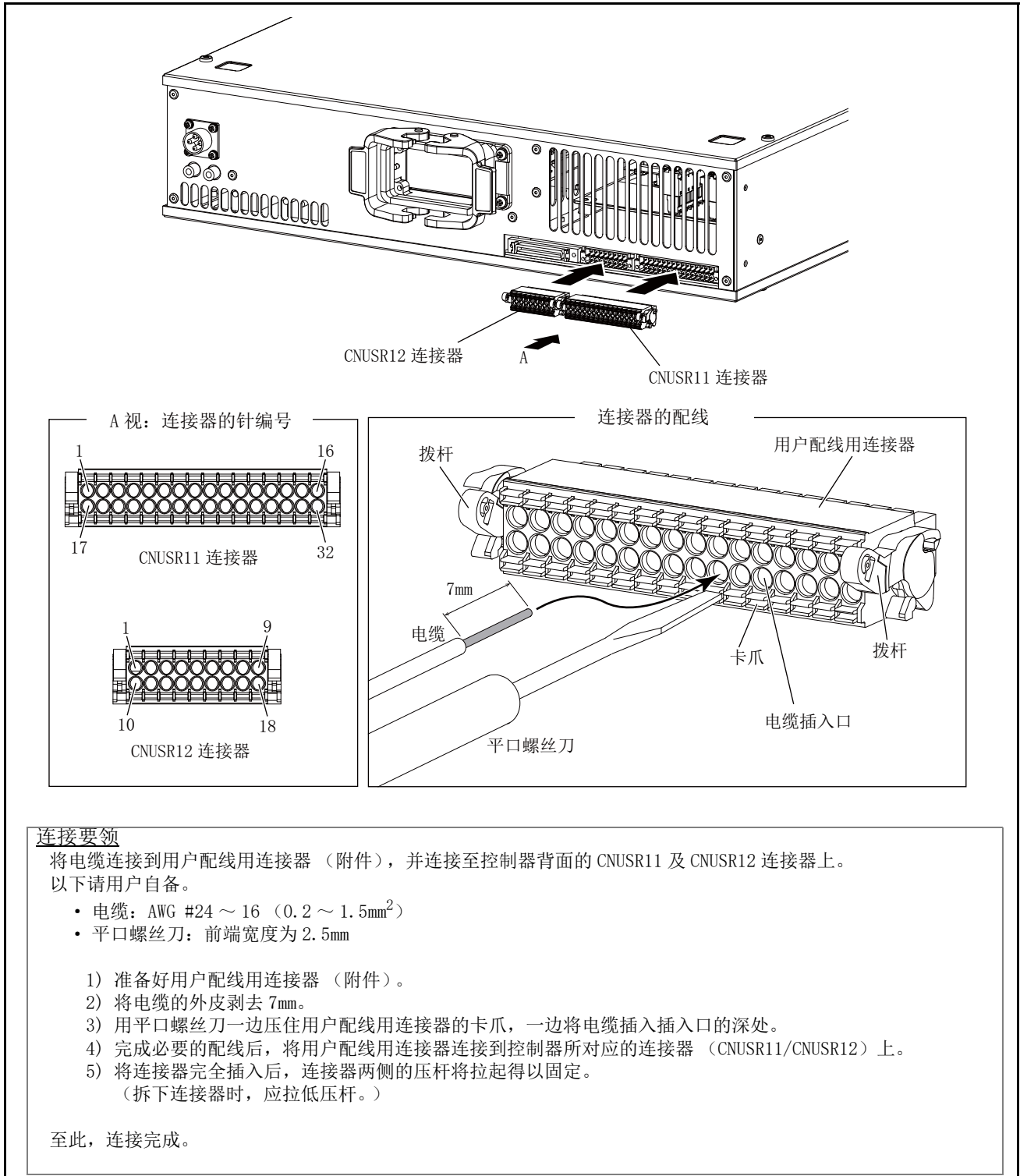
图 3-9：用户配线用连接器的配线方法
