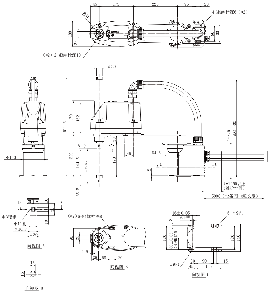
图 2-10: RH-3CRH4018 本体外形图
