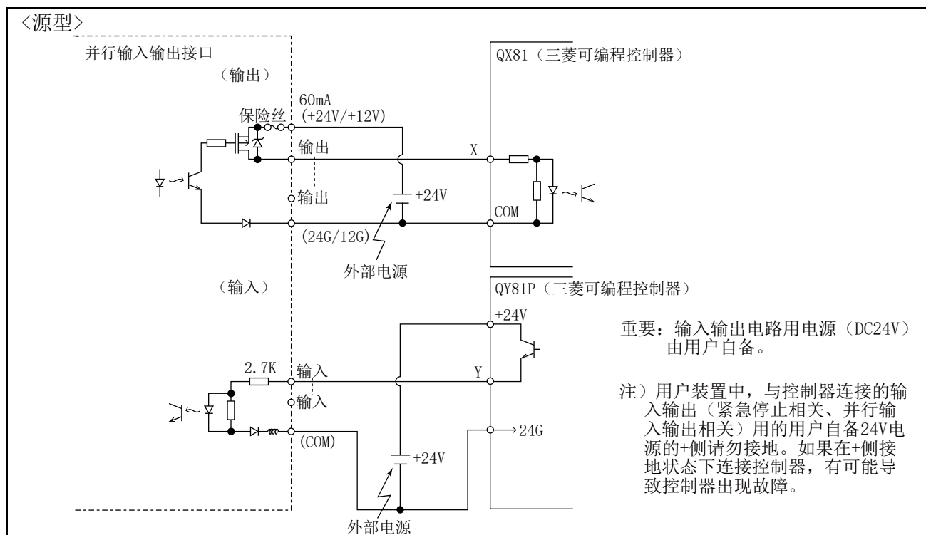
图 3-25：与三菱可编程控制器的连接示例（源型）
