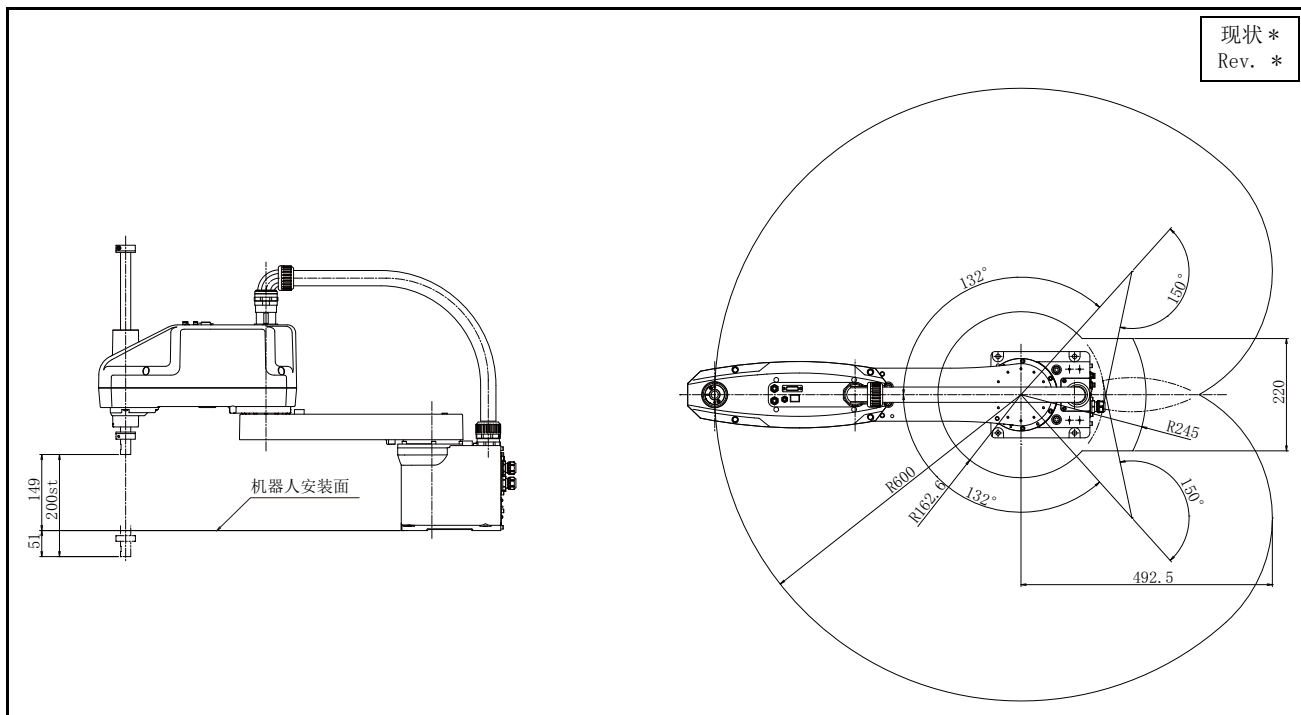
图 2-13: RH-6CRH6020 动作范围图
