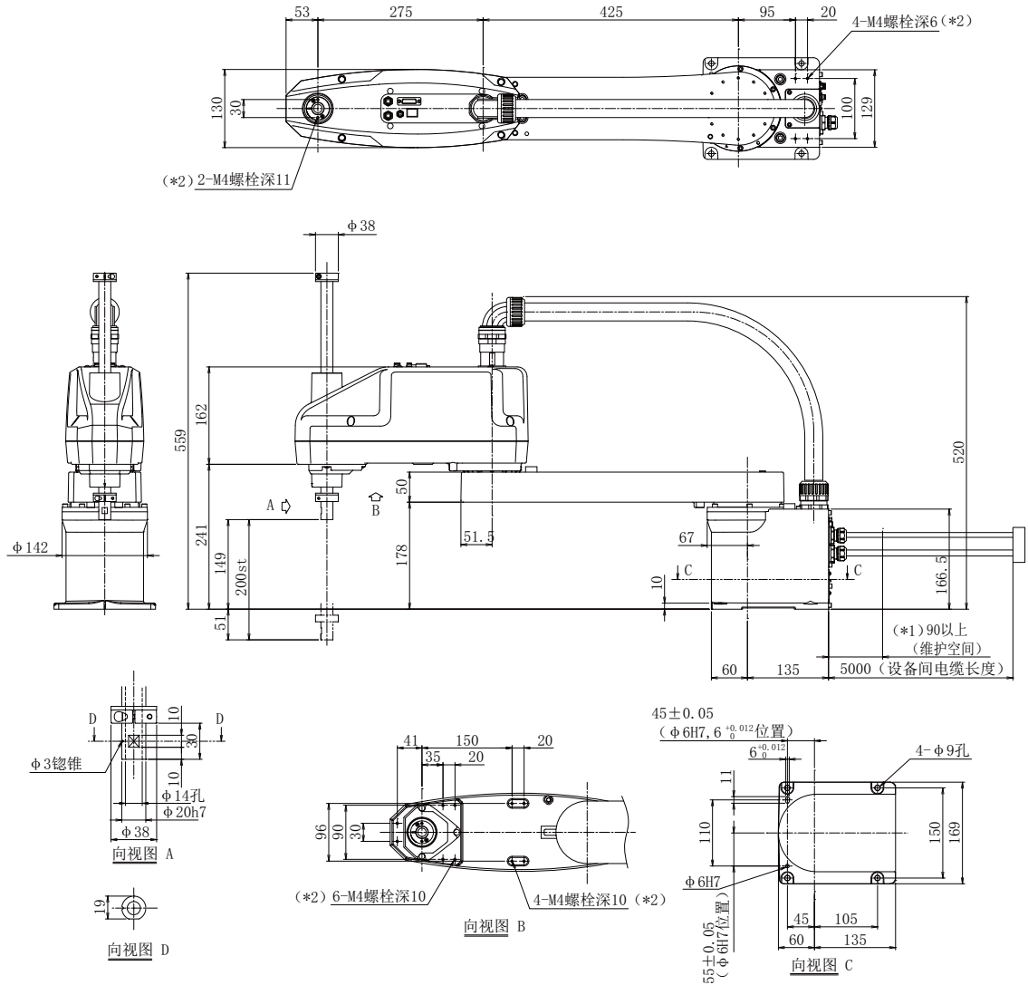
图 2-14: RH-6CRH7020 本体外形图
