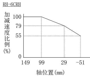
图 2-5: 加减速度的自动补偿
