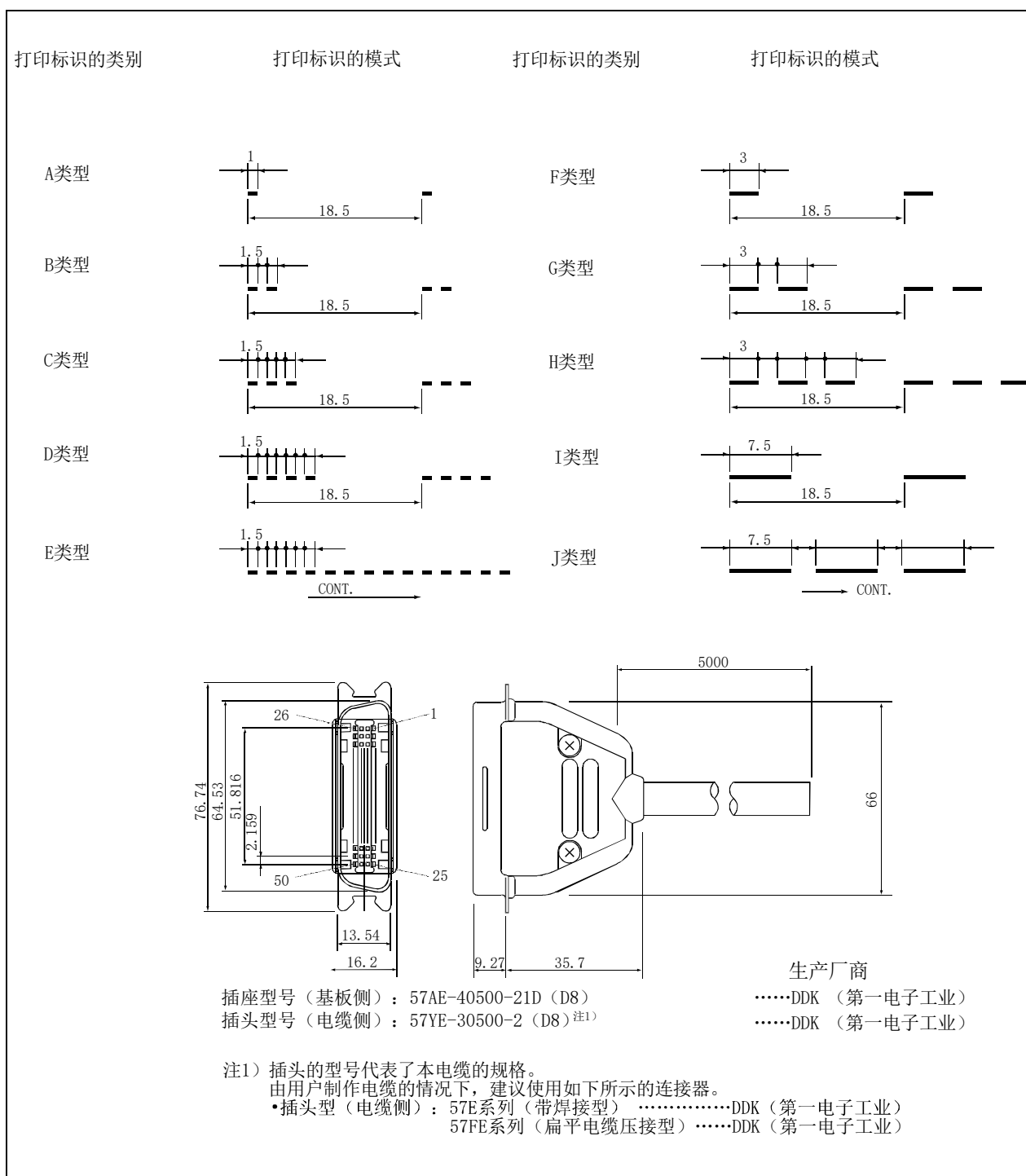
图 3-36: 连接 · 外形尺寸
