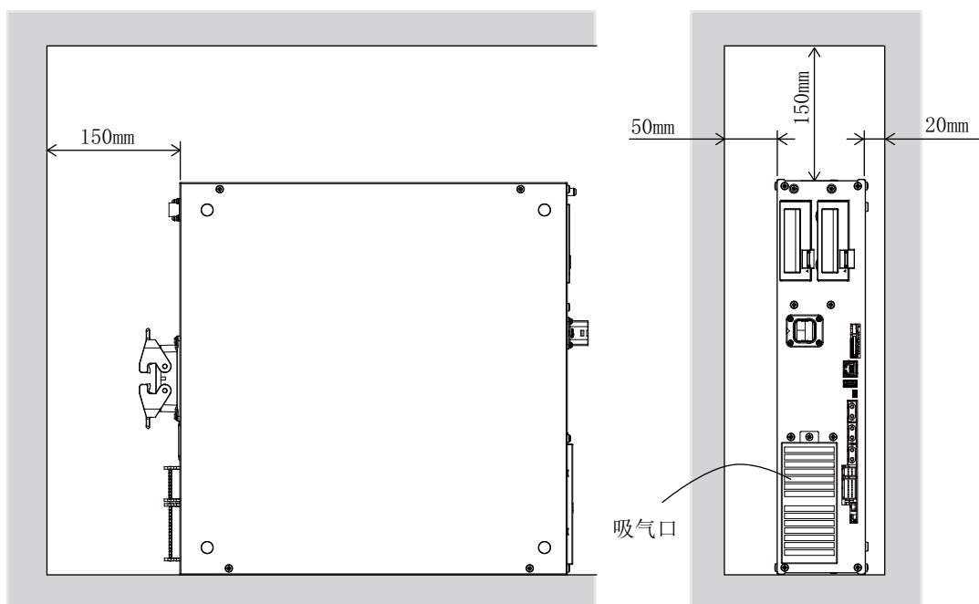
图 3-3: 安装尺寸
