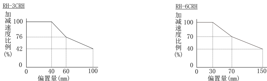
图 2-6：偏置量和最大速度的关系
