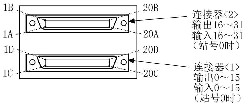
图 3-22：并行输入输出接口的连接器针配置
