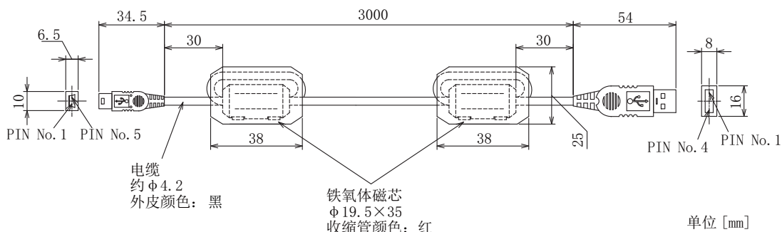
图 1-4: USB 电缆 (GT09-C30USB-5P)
