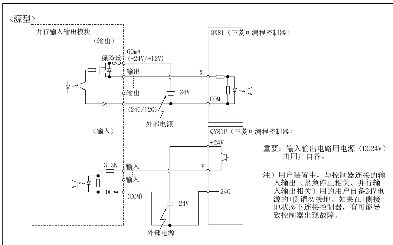
图 3-34：与三菱可编程控制器的连接示例（源型）
