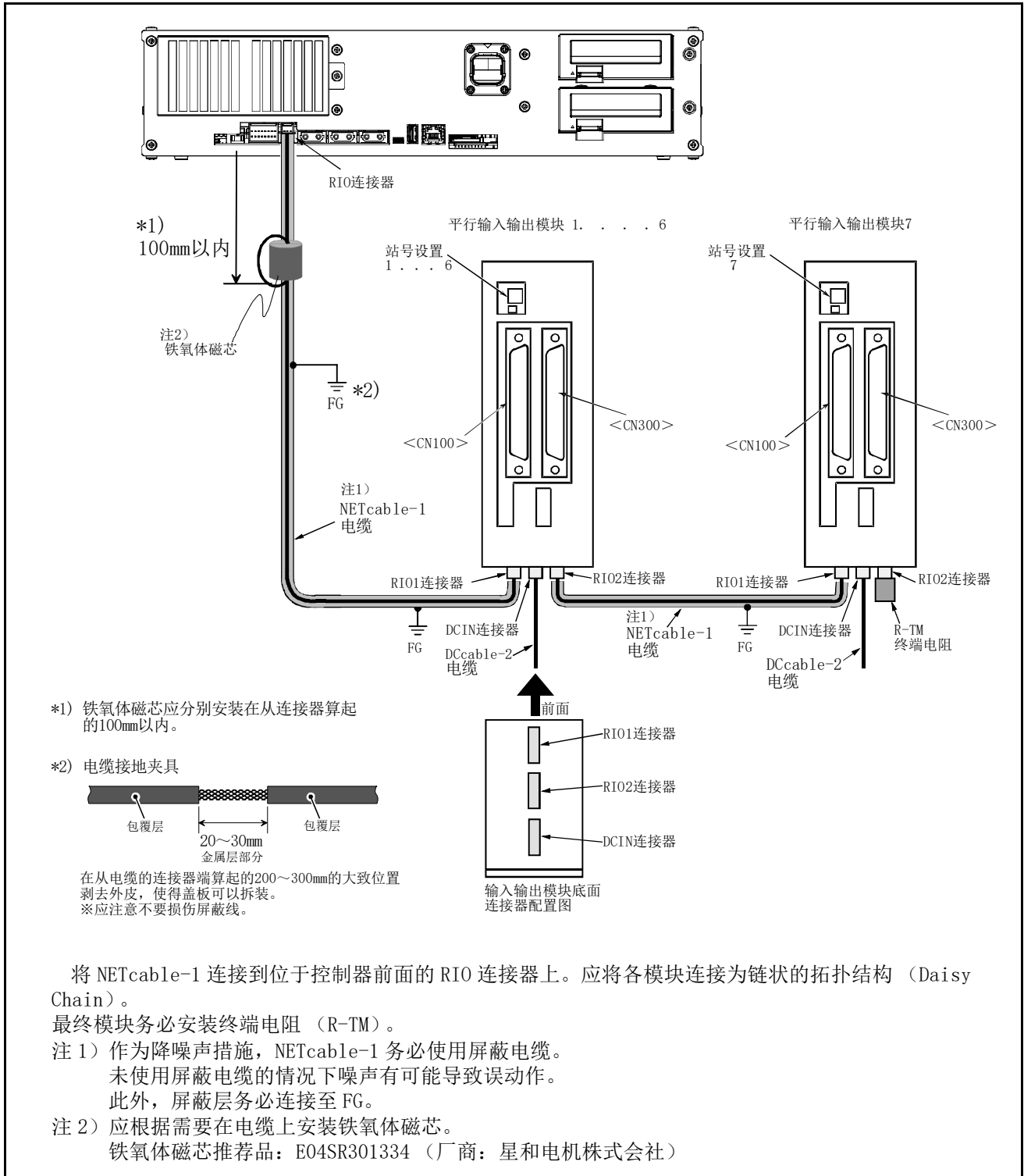
图 3-30：扩展并行输入输出模块的连接方法
