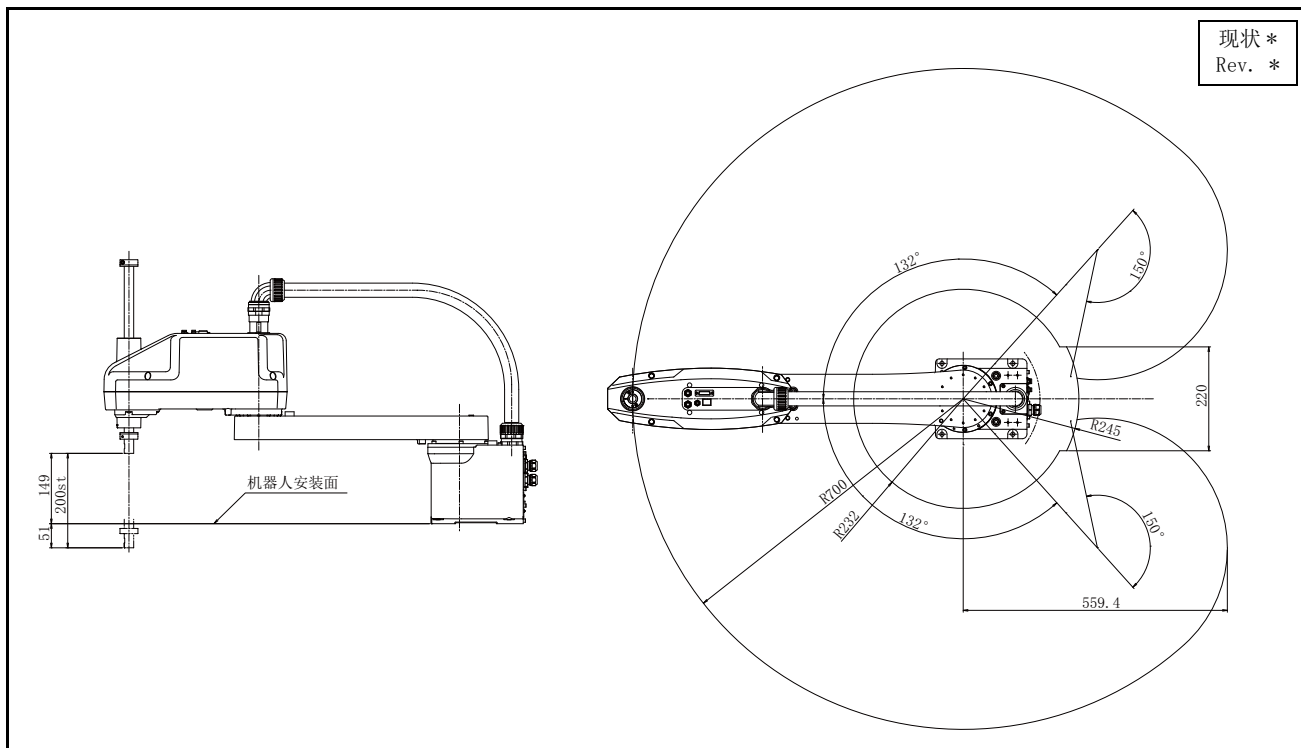
图 2-15: RH-6CRH7020 动作范围图
