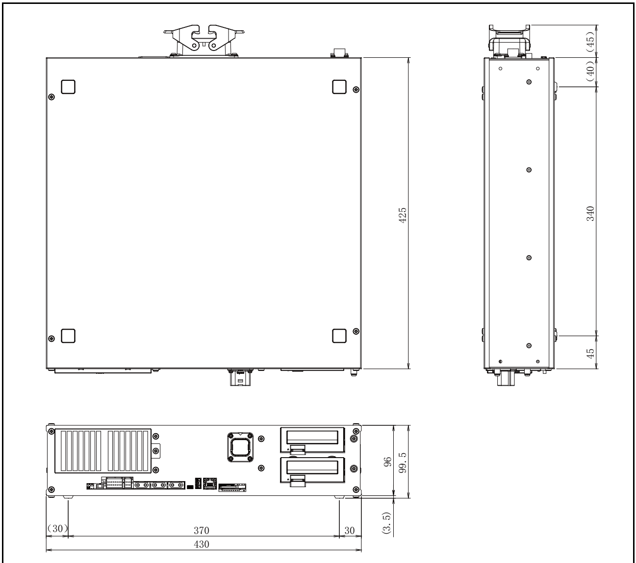
图 3-2：控制器的外形尺寸图
