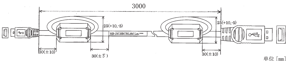
图 1-5: USB 电缆 (MR-J3USBCBL3M)
