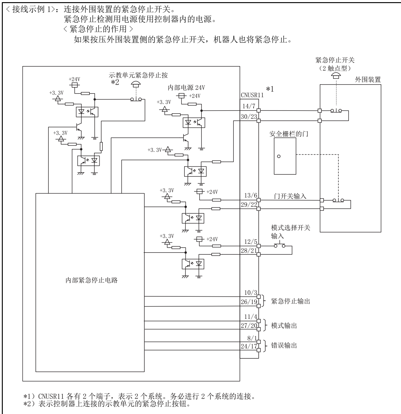
图 6-1：安全措施示例（配线示例 1）
