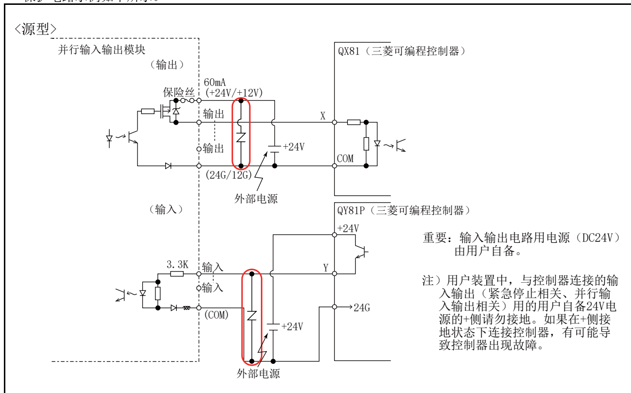
图 3-35：与三菱可编程控制器的连接示例（源型）保护电路示例
