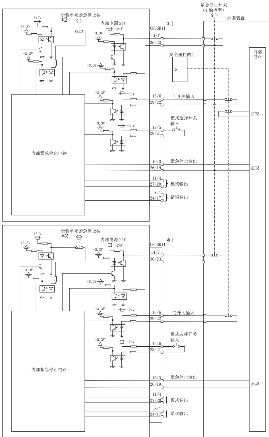
图 6-3：安全措施示例（配线示例 3）
