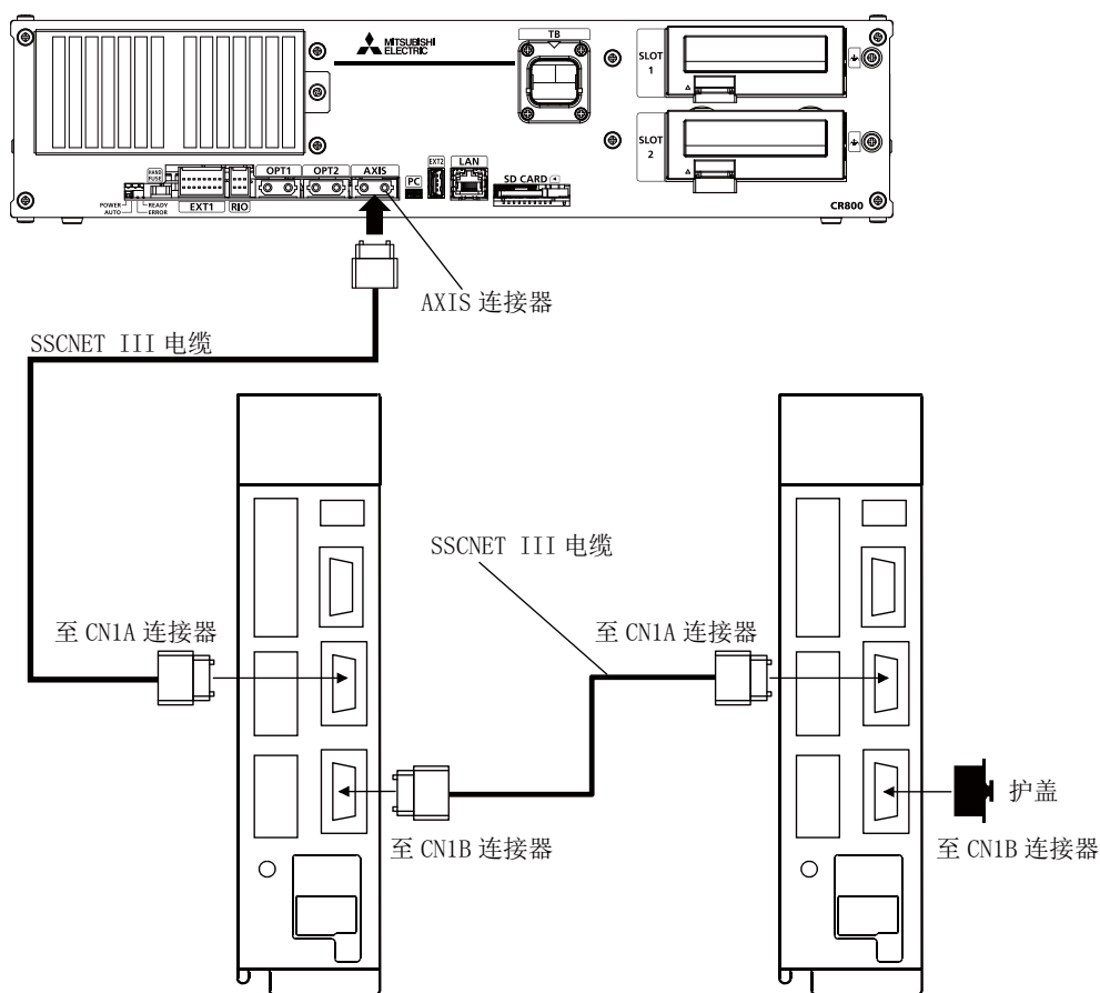
图 3-13：附加轴接口连接示例
