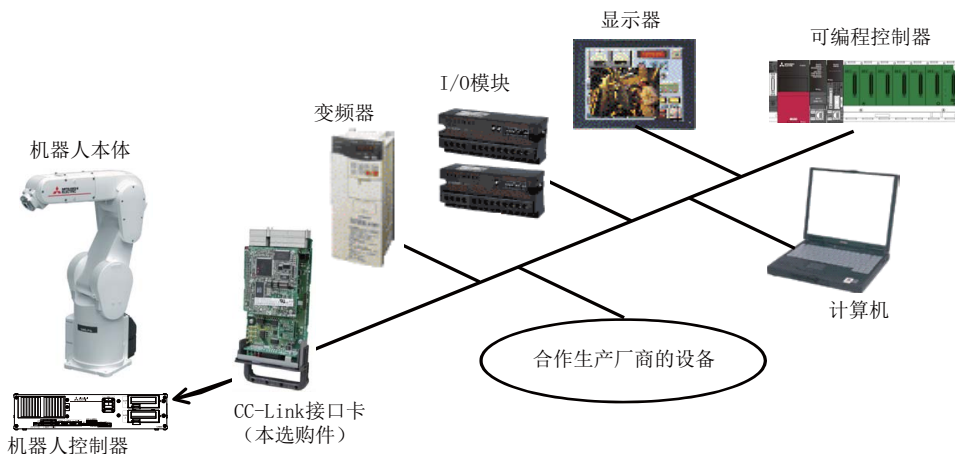
图 3-37：CC-Link 产品构成示例
