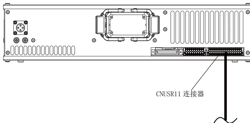
图 3-7：紧急停止电缆及模式选择开关的连接
