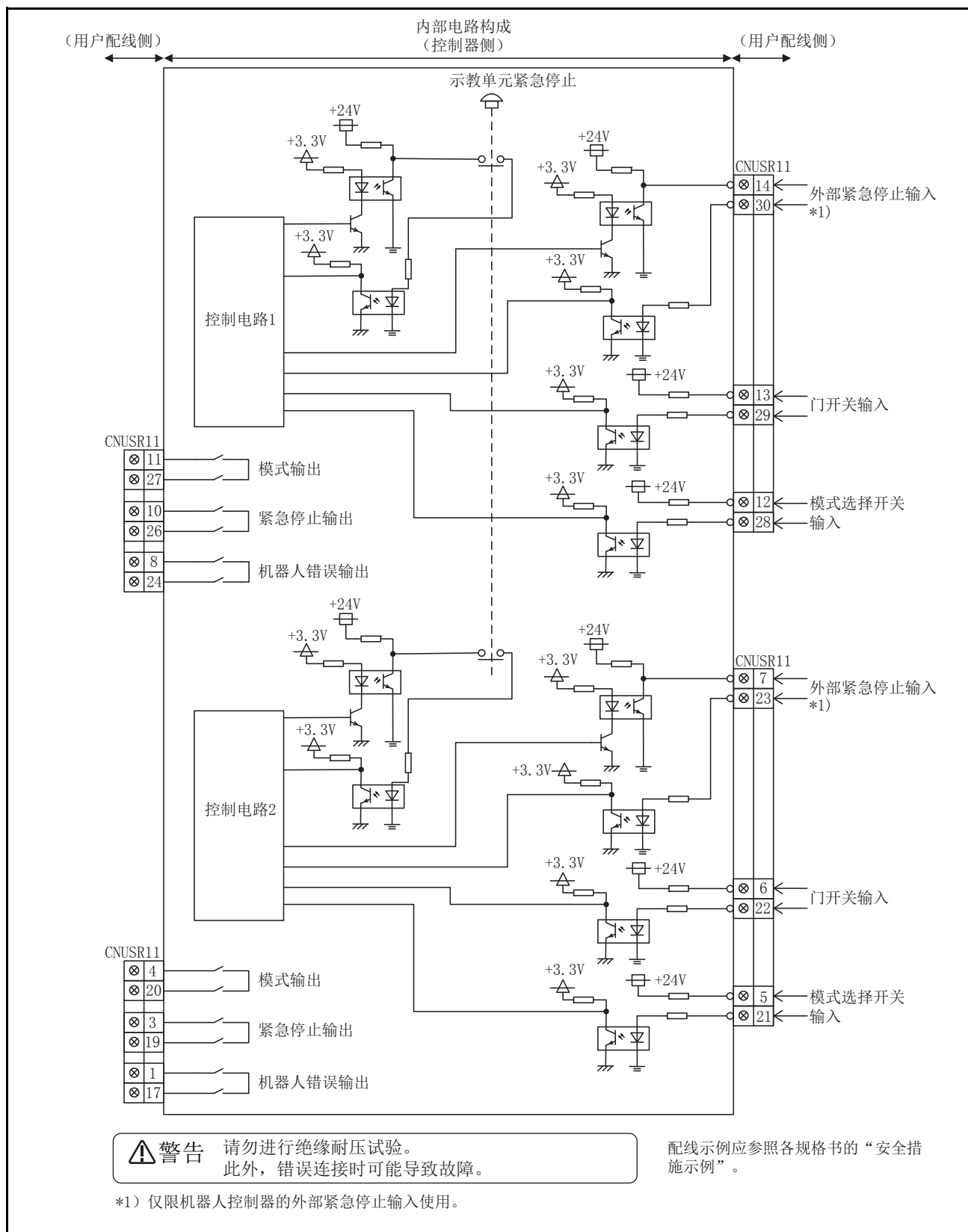
图 3-8: 外部紧急停止的连接
