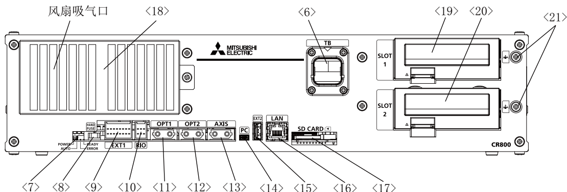
控制器前面
