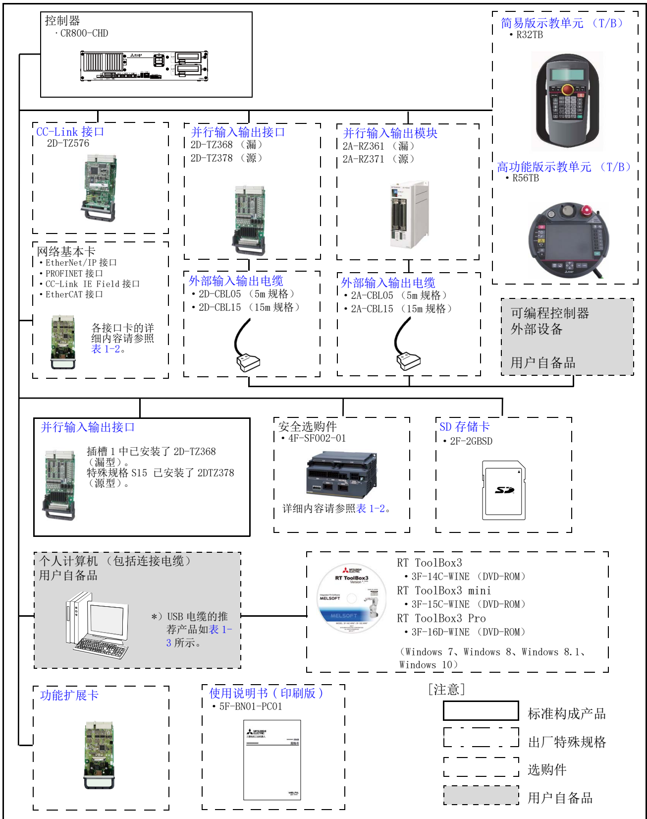
图 1-2: 构成设备的概要
