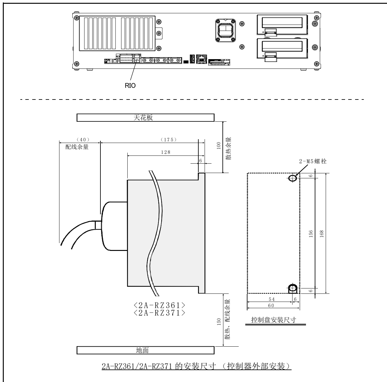
图 3-29: 并行输入输出模块安装方法
