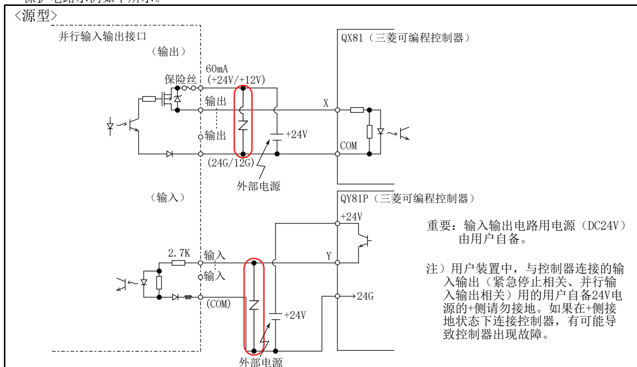
图 3-26：与三菱可编程控制器的连接示例（源型）保护电路示例
