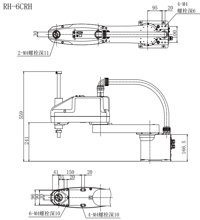
图 2-18: 配线配管固定用螺栓孔的位置 (RH-6CRH)
