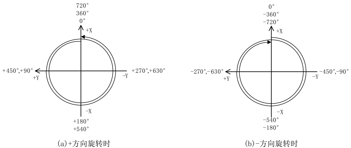
图 4-2: RH-3CRH/RH-6CRH 的 C 成分的定义 (超出 \pm 180^\circ 显示)
