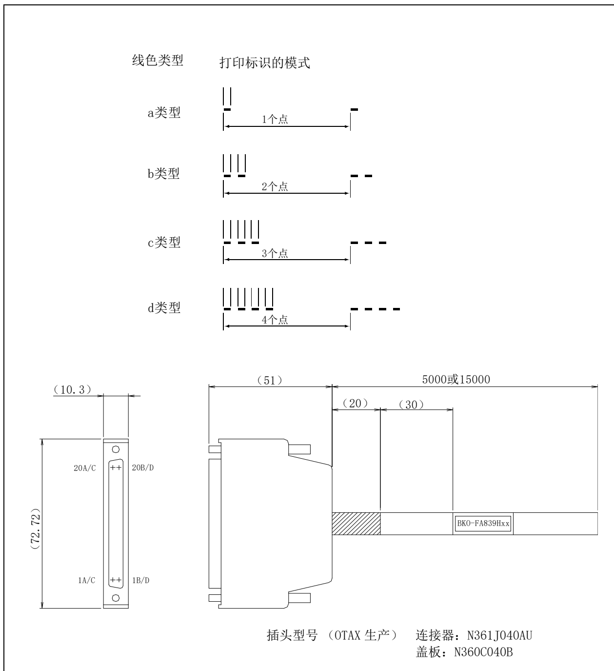
图 3-27: 连接 · 外形尺寸
