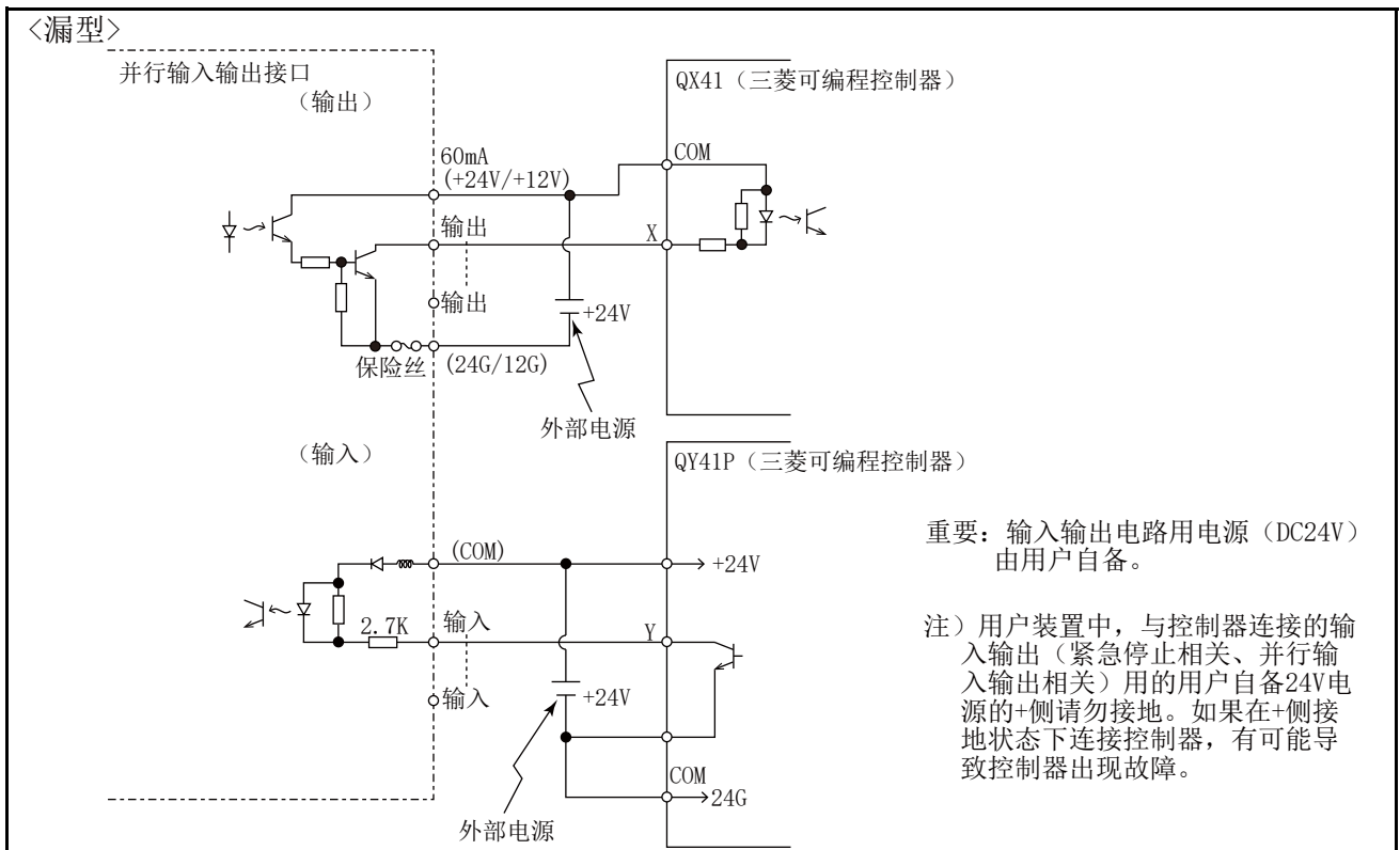
图 3-23：与三菱可编程控制器的连接示例 (漏型)
