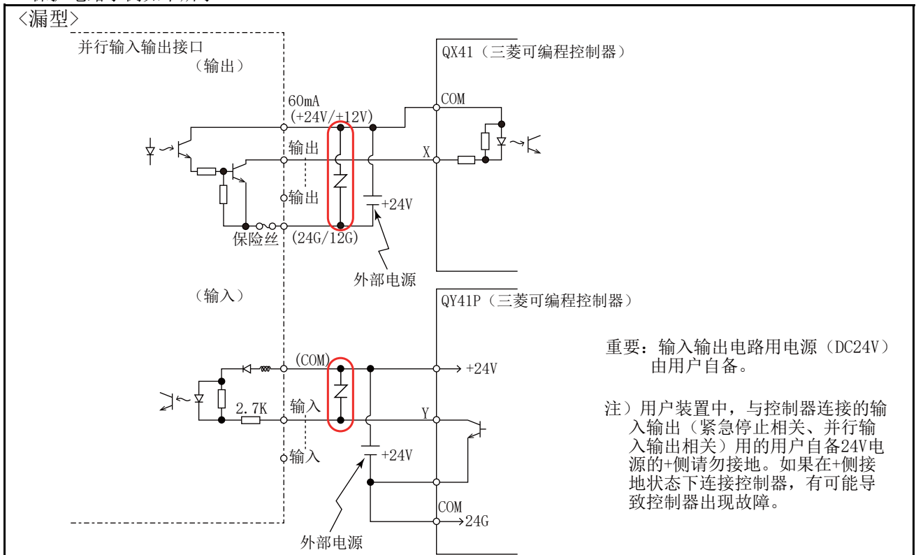
图 3-24：与三菱可编程控制器的连接示例 (漏型) 保护电路示例
