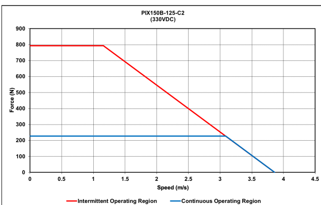
PIX150B-125-C2
