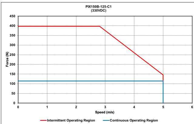
PIX150B-125-C1
