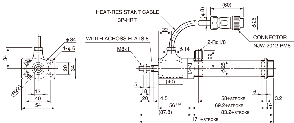
CSAH-20×□-FB
