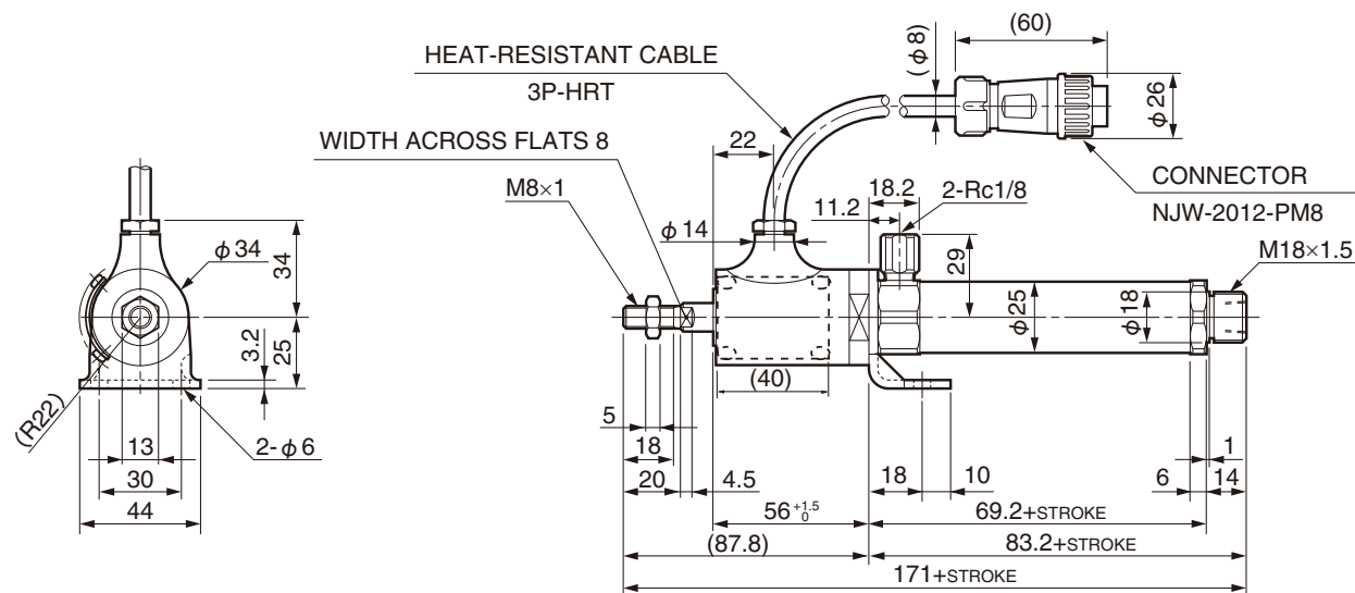
CSAH-20×□-LS
