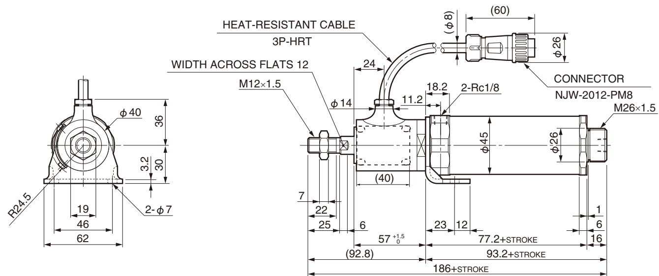
CSAH-40×□-LS
