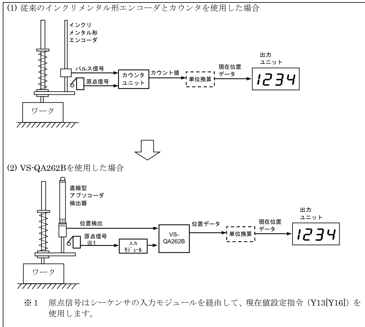
図1.1 現在値検出機能使用例
