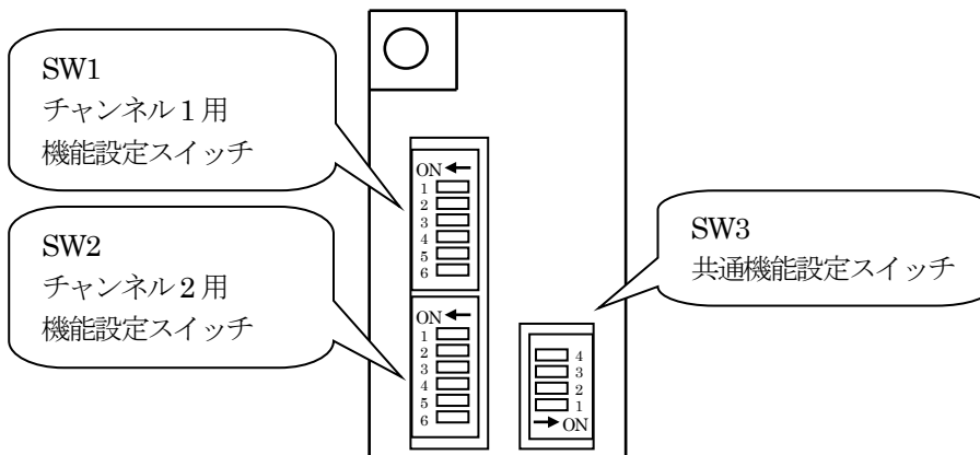
変換器 裏面
