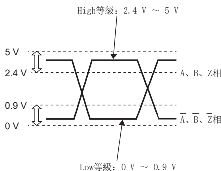
CN2L連接器連接點的伺服擴大器輸入訊號等級
