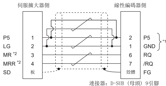
連接器：D-SUB（母頭）9引腳
