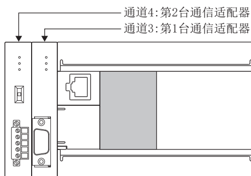
[构成例2]
