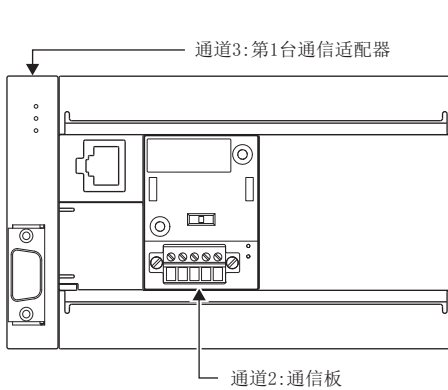
[构成例1]
