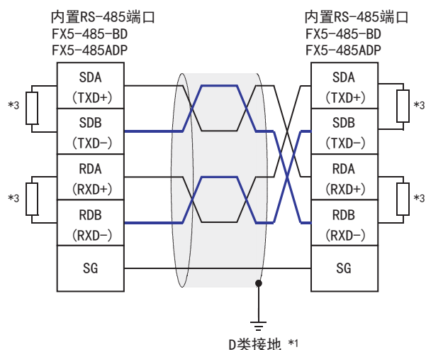
■2对接线
