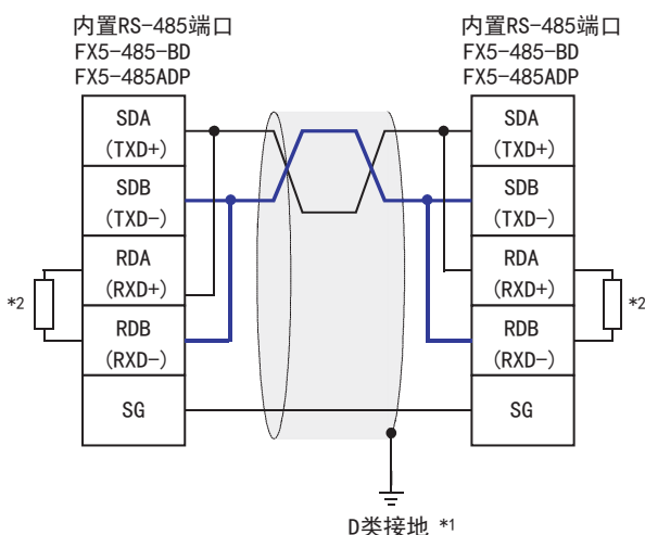
■1对接线
