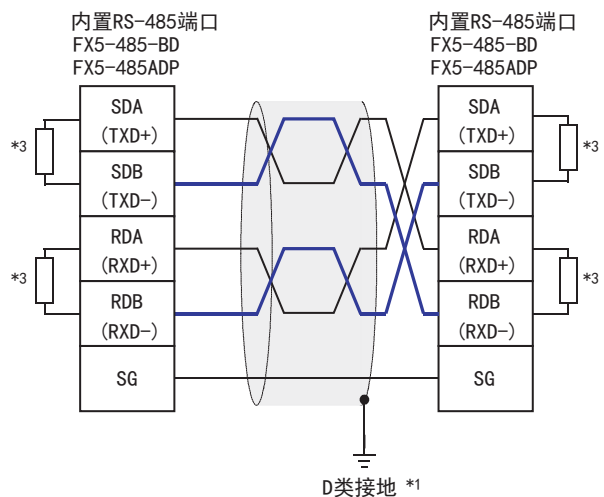
■2对接线
