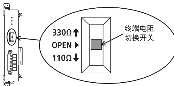
■FX5-485ADP
