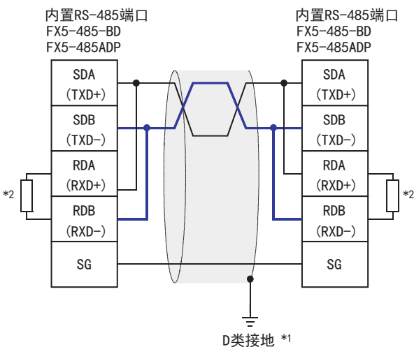
■1对接线
