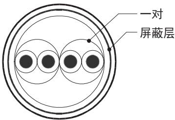
2对电缆的结构图例
