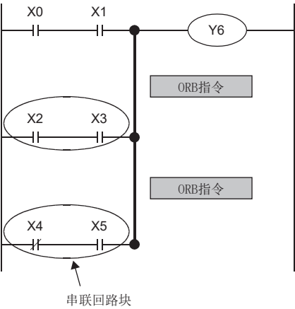
回路程序
