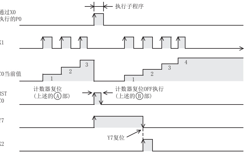
时序图
