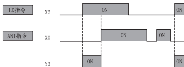
时序图
