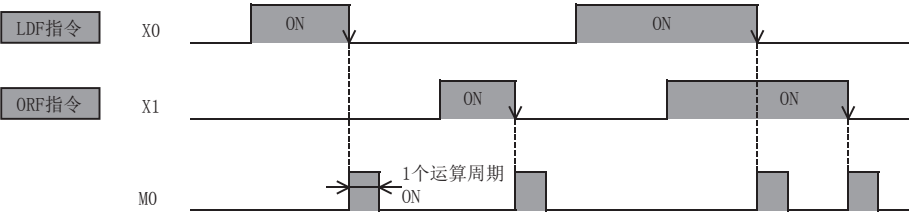
时序图
