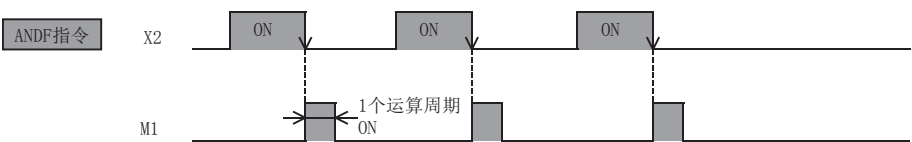
时序图
