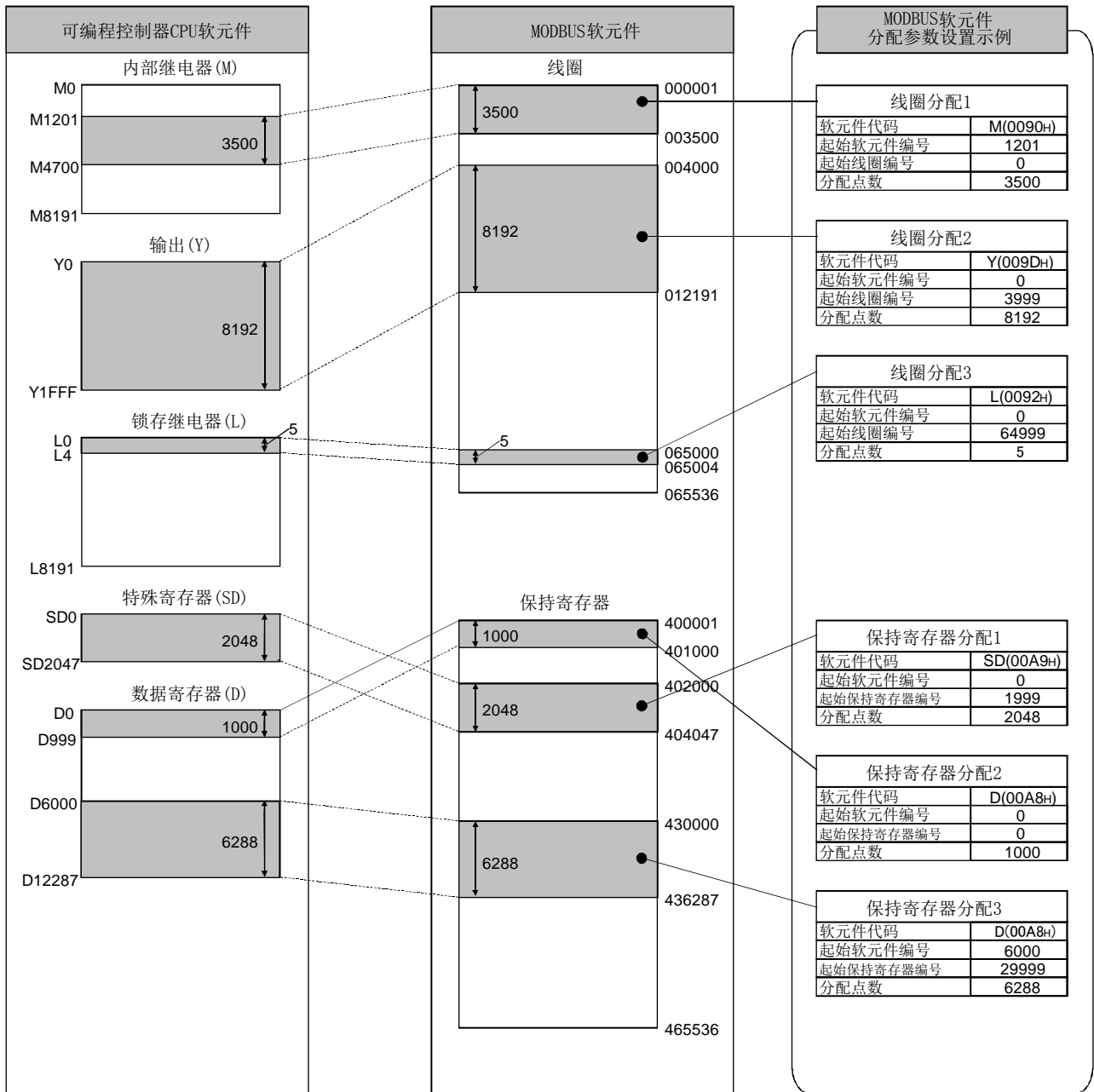
[MODBUS软件元件分配参数的设置示意图]
