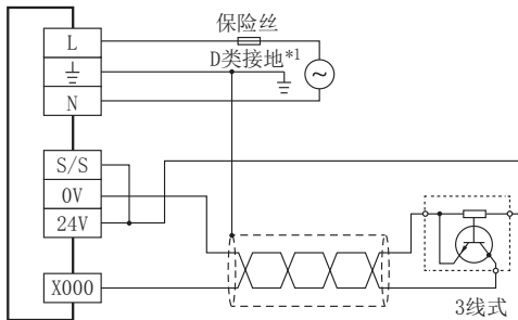
漏型接线的场合
