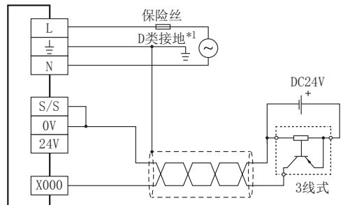
源型接线的场合
