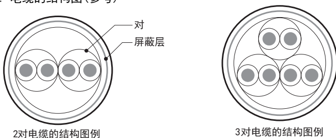
2对电缆的结构图例
