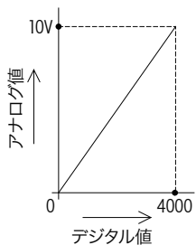
電圧出力特性(0~10V) 工場出荷時特性
