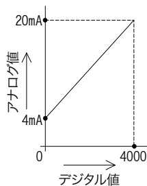
電流出力特性(4~20mA)
