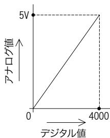
電圧出力特性(0~5V)
