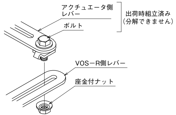
図3 レバーの連結2
