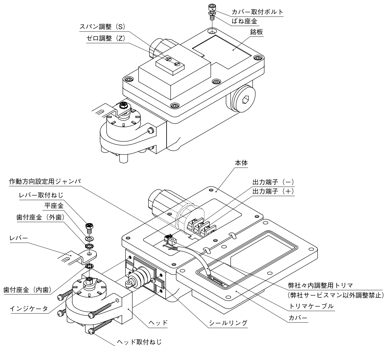
図1 各部の名称
