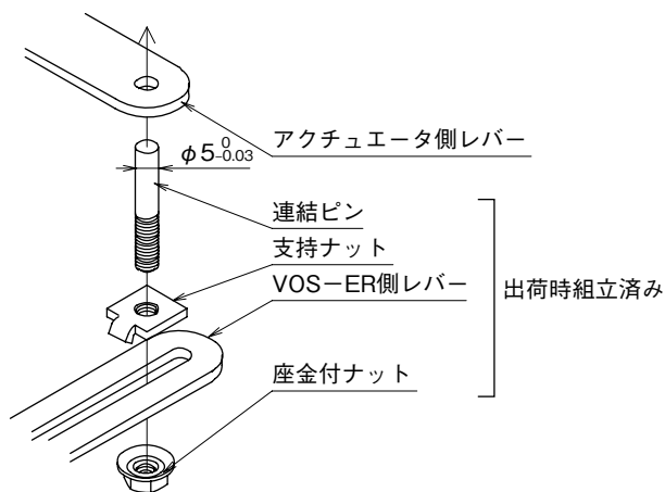
図2 レバ－の連結1
