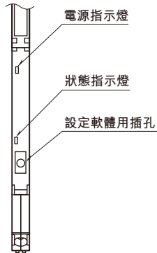
■ 前視圖 (上蓋打開時)
