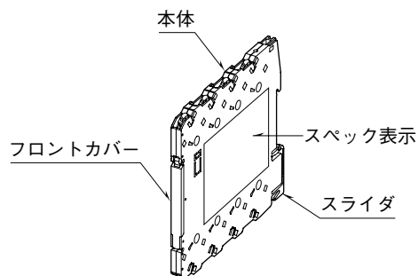
■前面図 (開蓋時)
