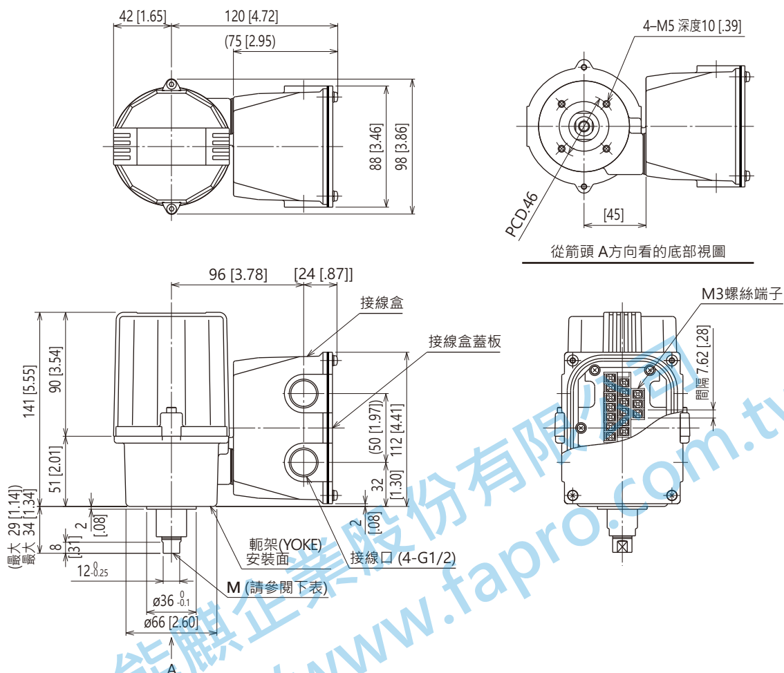
出力軸形狀 M
