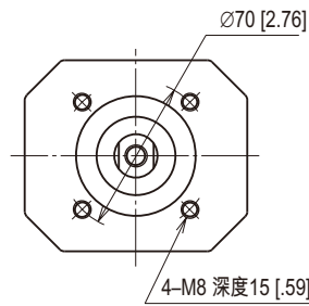
軛架(YOKE) 安裝尺寸圖
