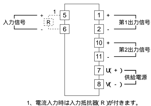
端子接続図
