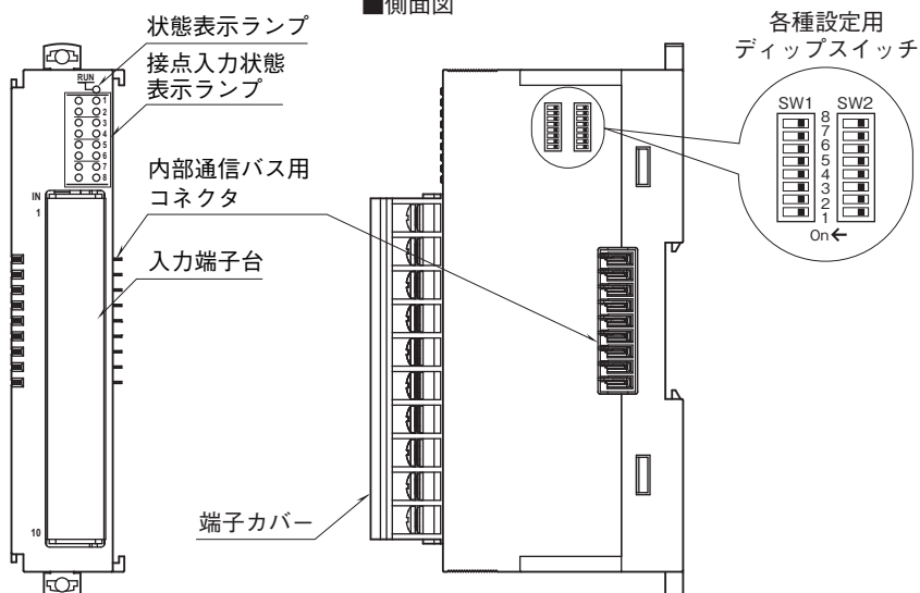
■側面図
