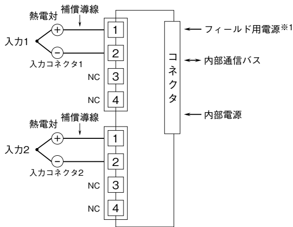
端子接続図
