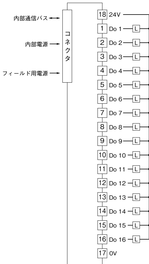
端子接続図
