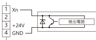
■ 2線式傳感器連接時
