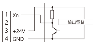
■ 3線式傳感器連接時
