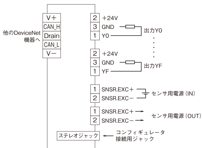
端子接続図
