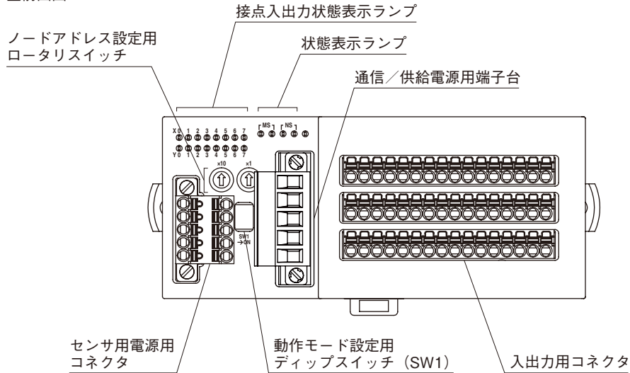
■前面図
