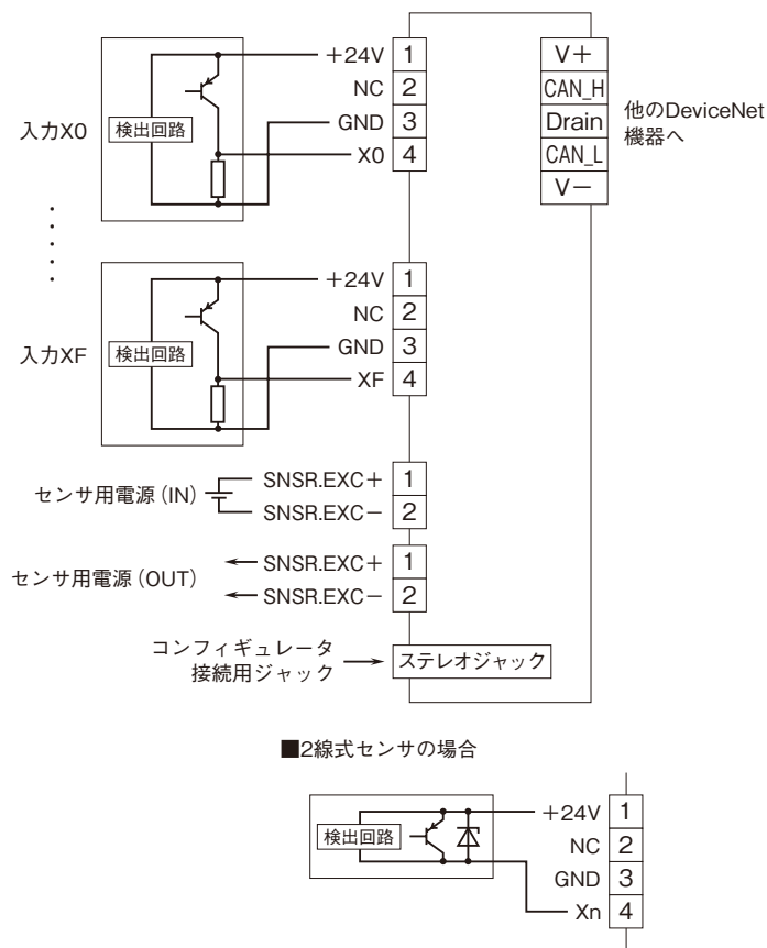
端子接続図
