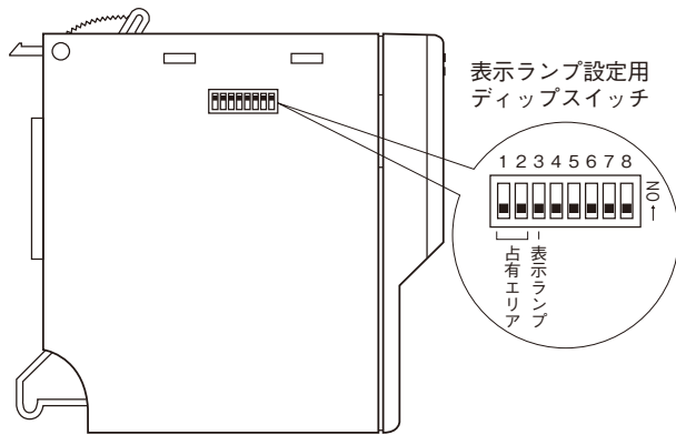
■側面図
