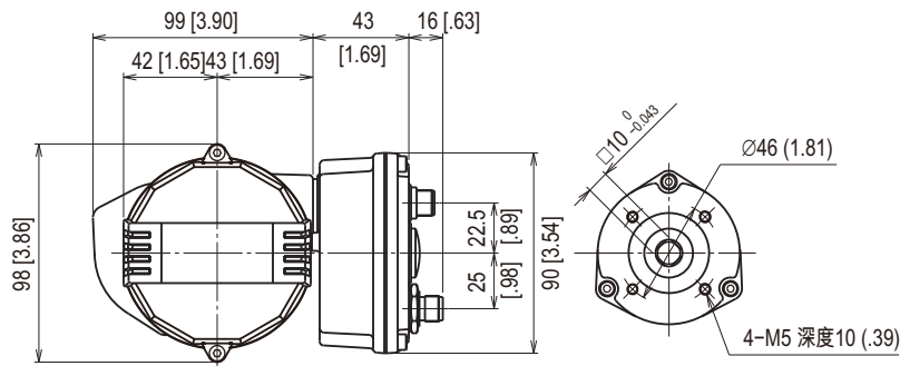
軛架(YOKE)安裝尺寸
