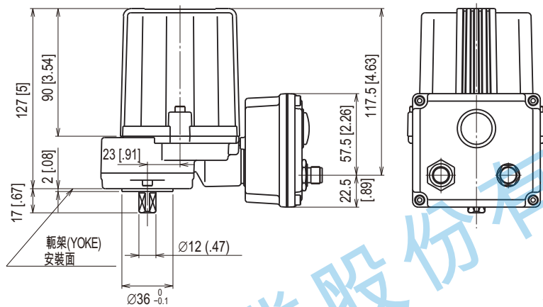
軛架(YOKE)安裝尺寸
