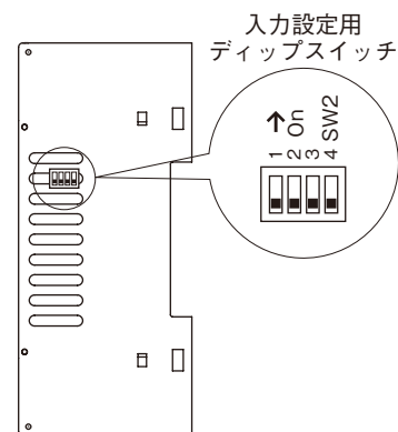
■右側面図
