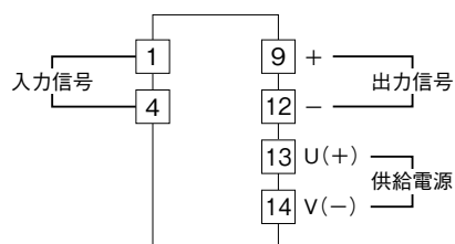
端子接続図
