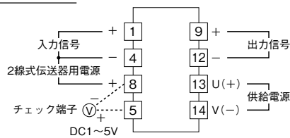
端子接続図
