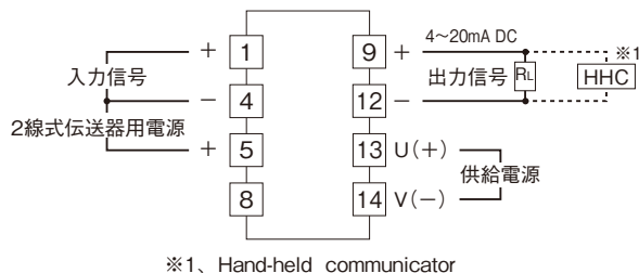
端子接続図
