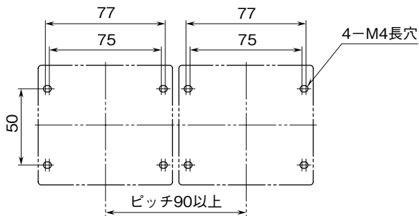
取付寸法図 (単位: mm)
