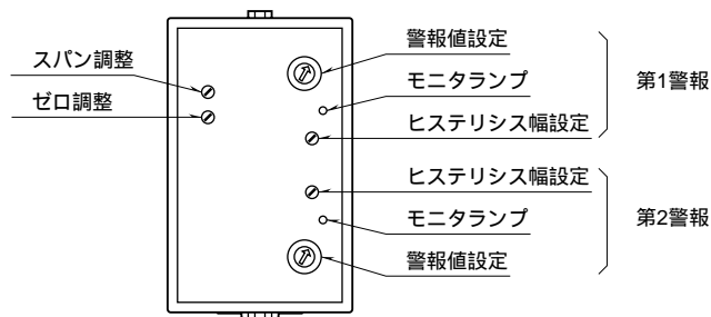
前面図
