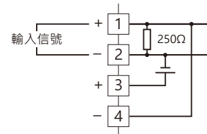
■ 4 ~ 20mA 直接輸入時
