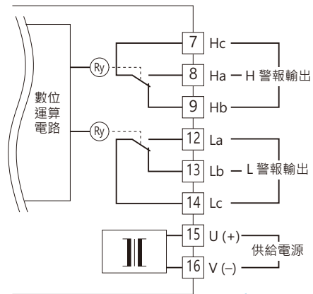
■ 警報輸出點數代碼 2: 2點
