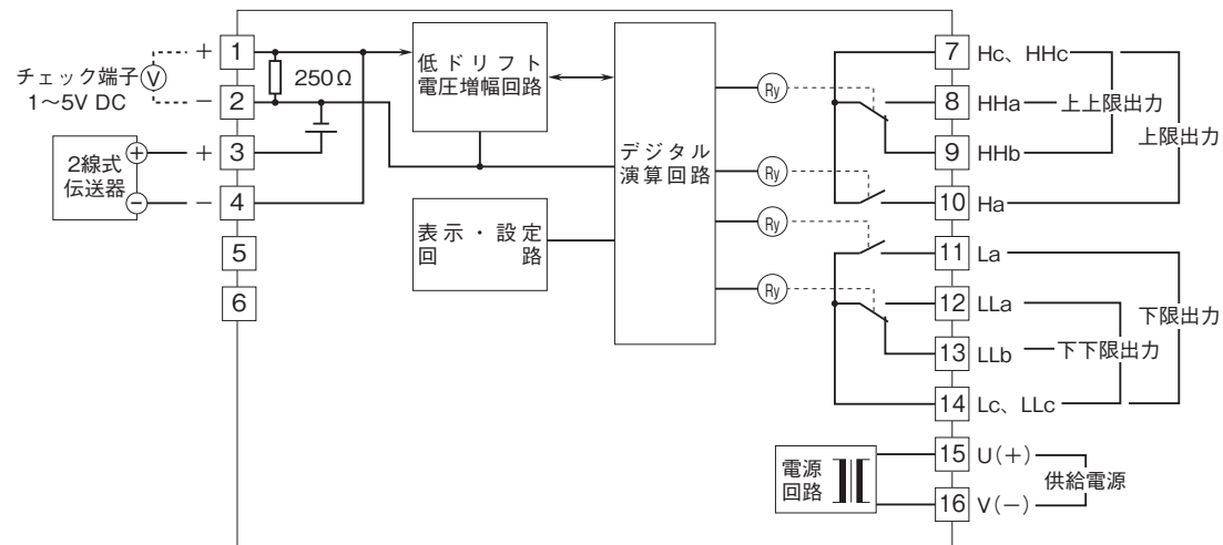
■48NAVD-4 (4点警報/4接点出力)
