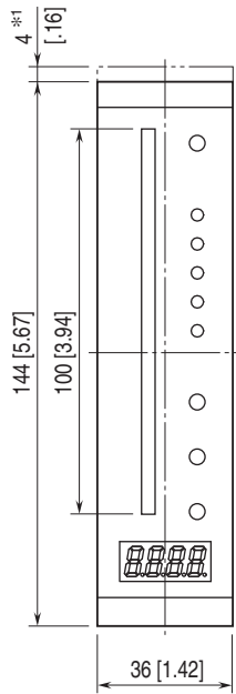
■ STANDARD BEZEL *2
