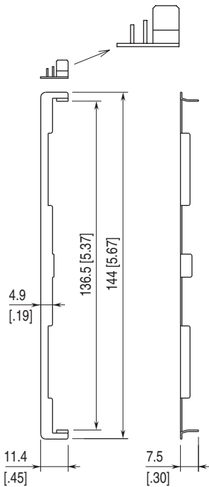
■ STANDARD BEZEL *2
