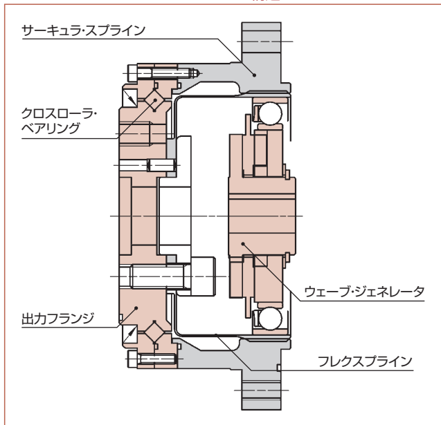
CSG/CSFシリーズユニットタイプの構造
